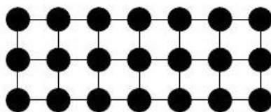
Obr. 2. Mriežkový graf ( 7 \times 3 ).
